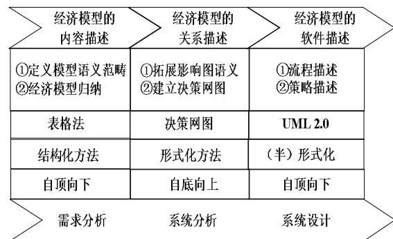
图 1 经济模型驱动的仿真建模方法
