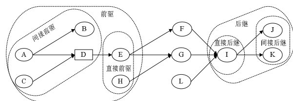
图 2 影响图的基本术语定义
