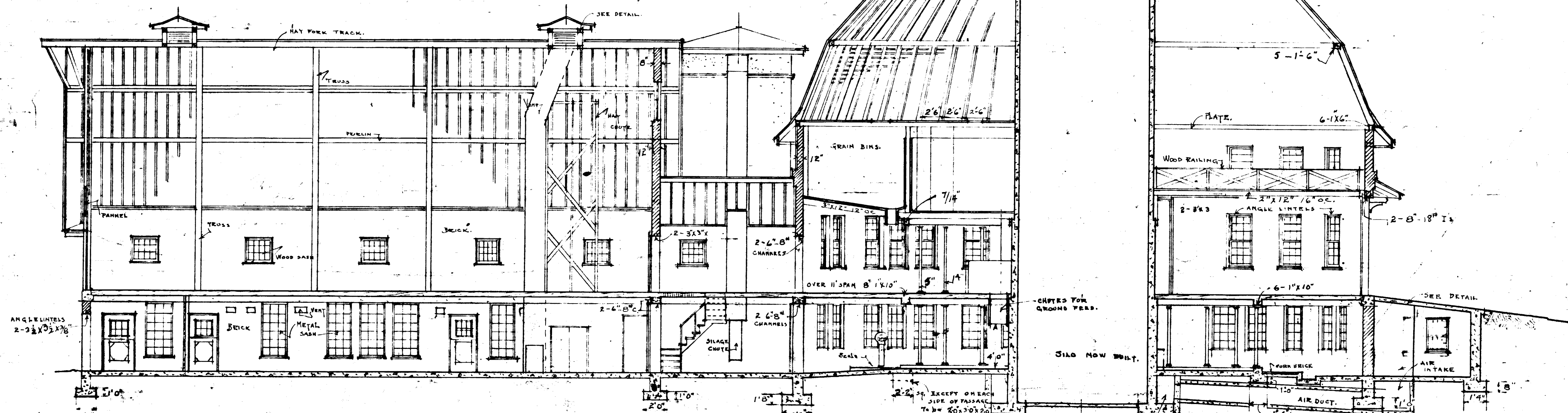
LONGITUDINAL SECTION Scale - 1/2" = 1'-0"
