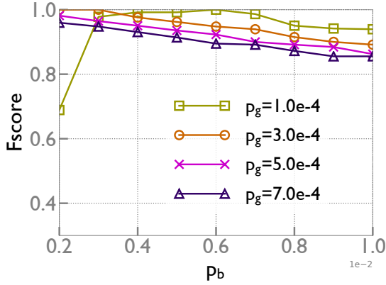
(a) Parameter sensitivity
